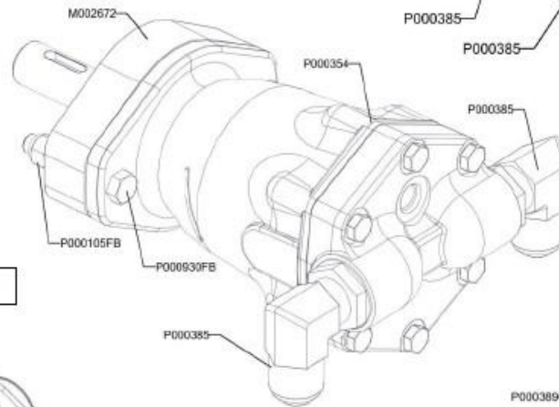
FAN MOTOR
